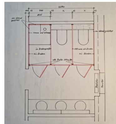
Plan vom WC und der Dusche
