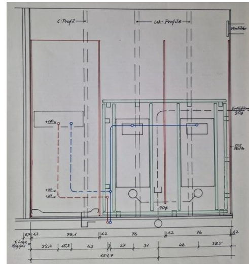
Plan der Leitungen und GIS-Profil
