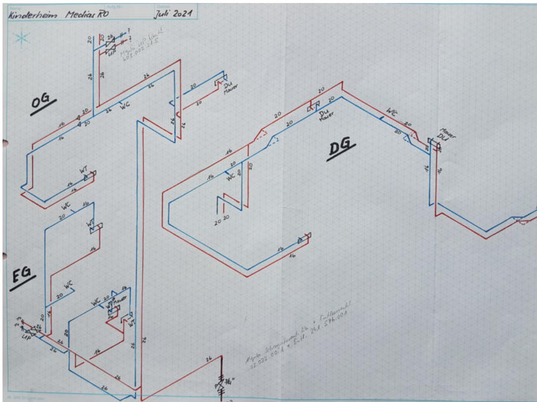
Plan der Warm- und Kaltwasserleitungen über die drei Geschosse.
