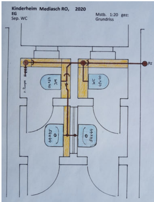
Plan 1 EG: Zwei separate WCs mit Lavabos.
