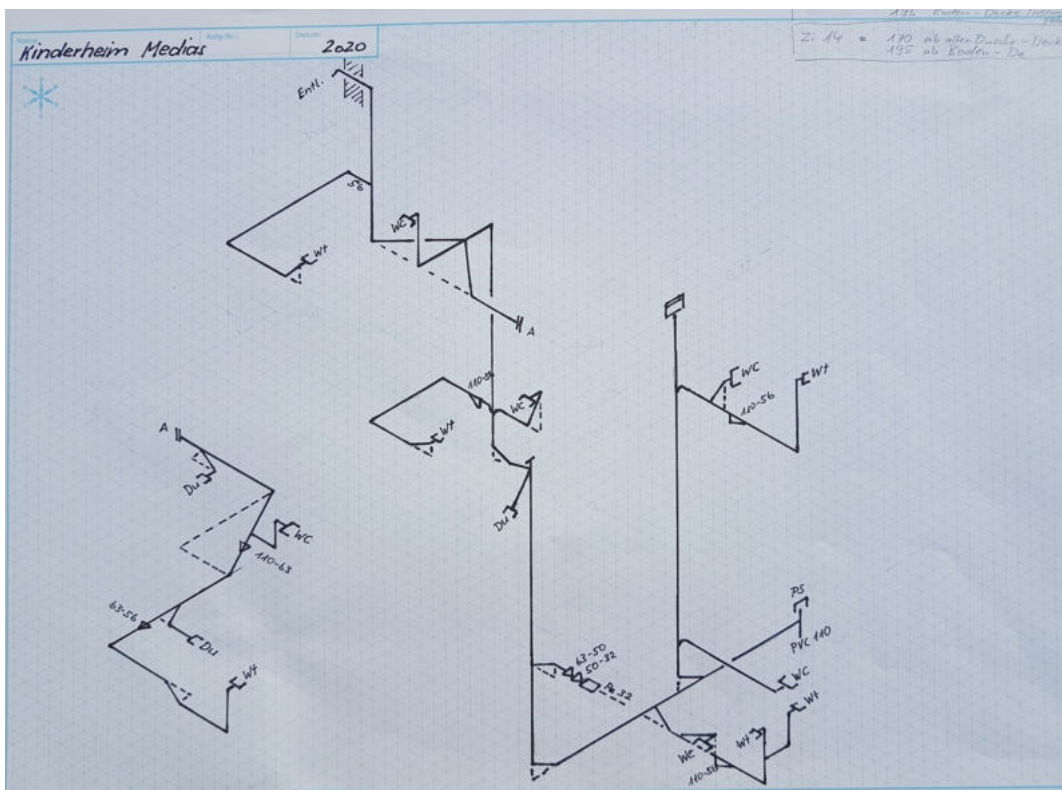
Plan der Abwasserleitungen über die drei Geschosse.
