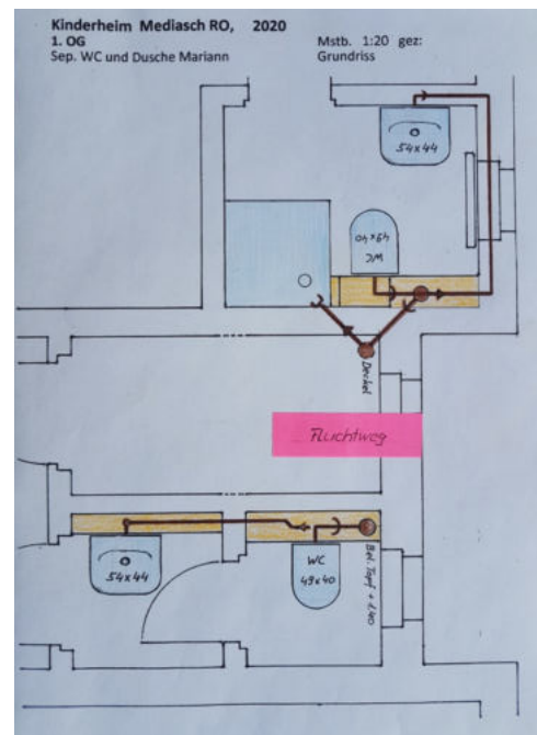
Plan 2 1. OG: Dusche mit WC und Lavabo in Marianns Zimmer, Fluchtweg und separates WC mit Lavabo.
